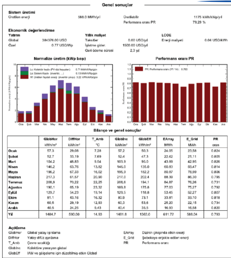
Projenin yerleşim alanına göre ışınlama analizi yapılarak sistemin üretim verimliliği ölçülür.
